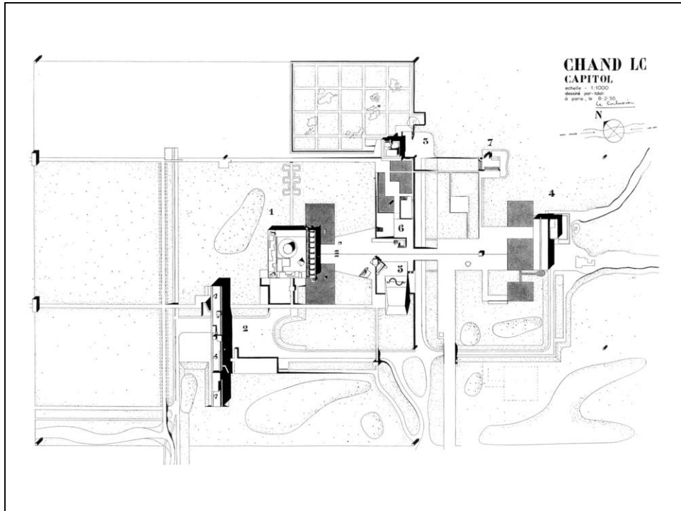
Le Corbusier, Planimetria del campidoglio di Chandigar, 1956 (1 Assemblea Generale; 2 Segretariato; 3 Palazzo del Governatore; 4 Alta Corte; 5 Torre dell'Ombra; 6 Martirium; 7 La Mano Aperta)
