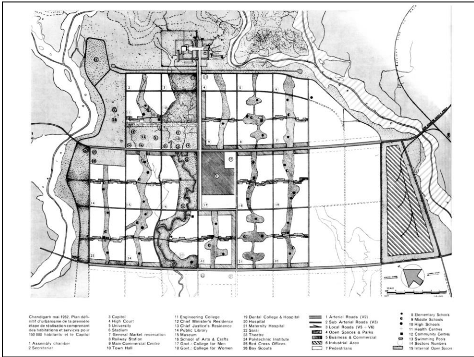
Le Corbusier, Piano generale per Chandigar, 1952
