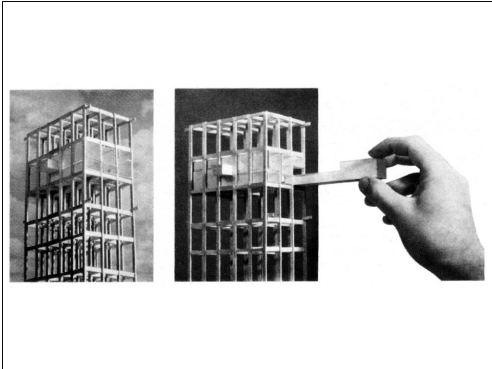
Le Corbusier, Il concetto del portabottiglie applicato all'Unité d'habitation, Marsiglia, 1945-1952
