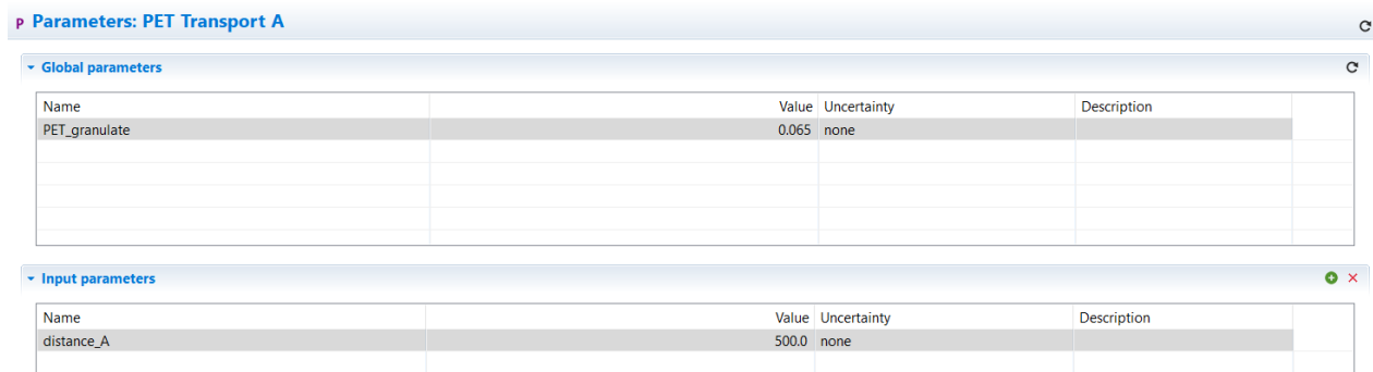
Figure 8.5: Parameters tab
