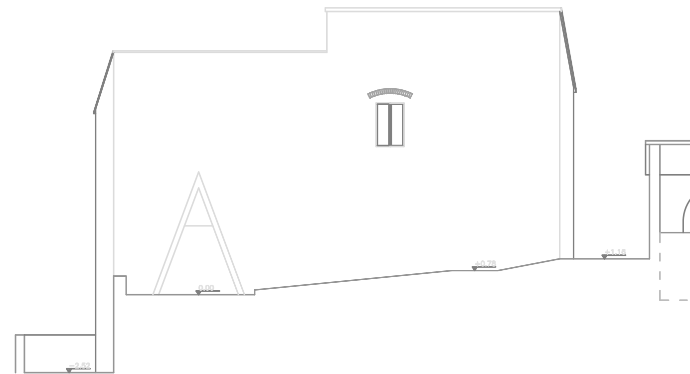
SEZIONE D-D
