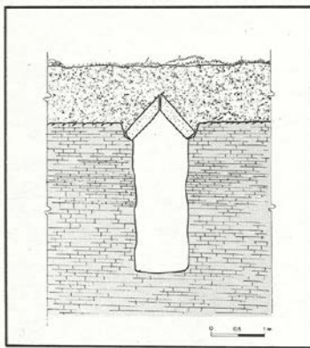
Fig. 15 - Caratteristica sezione trasversale del qanat di Castelforte (Partanna Mondello) che con i suoi 1400 m di lunghezza attraversa la piana dei Colli. La copertura è realizzata «a bocca di forno» con due conci di tufo inclinati a doppio spicciante.
