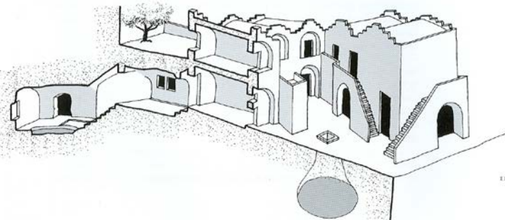
68. Vicinato. Pianta e sezione
