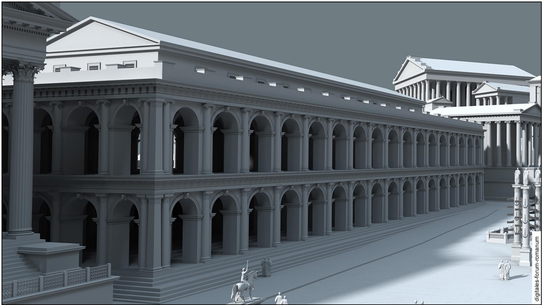
Basilica Julia, Roma, I sec. a.C. (ricostruzione)
